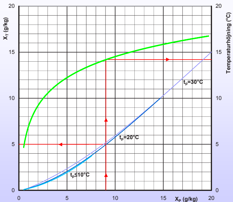
KAPACITETSDIAGRAM
