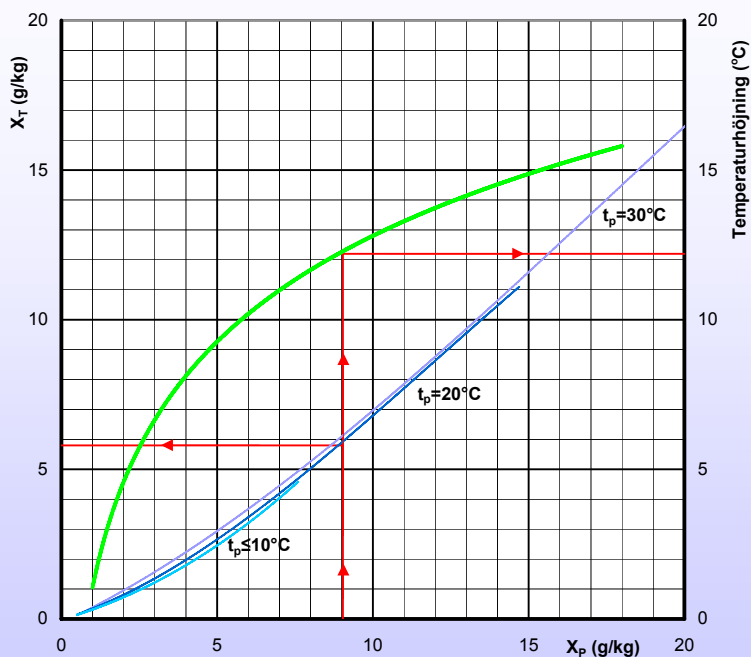
KAPACITETSDIAGRAM
